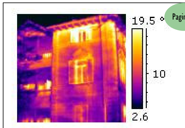
Esempio di termografia del municipio di pecetto
